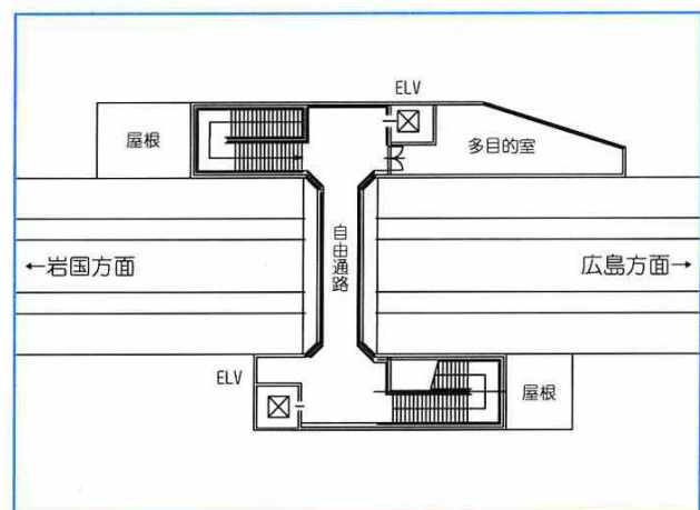
駅2階平面図
