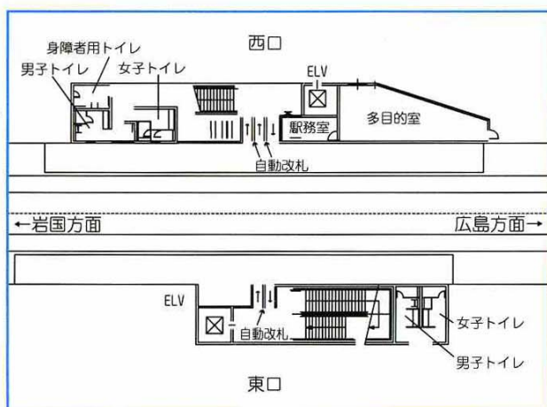
駅1階平面図
